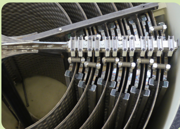
Agencement des brosses de nettoyage
