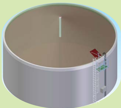
farmAS® - Fosse de stockage ronde en béton armé - Vue du haut
